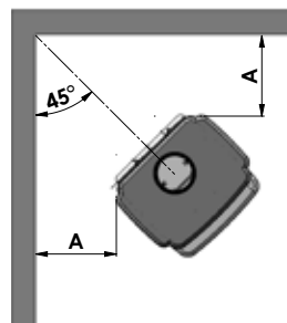
3440 hoekinstallatie
