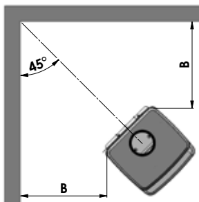
3410/3450 hoekinstallatie
